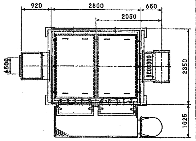
A矢視図
